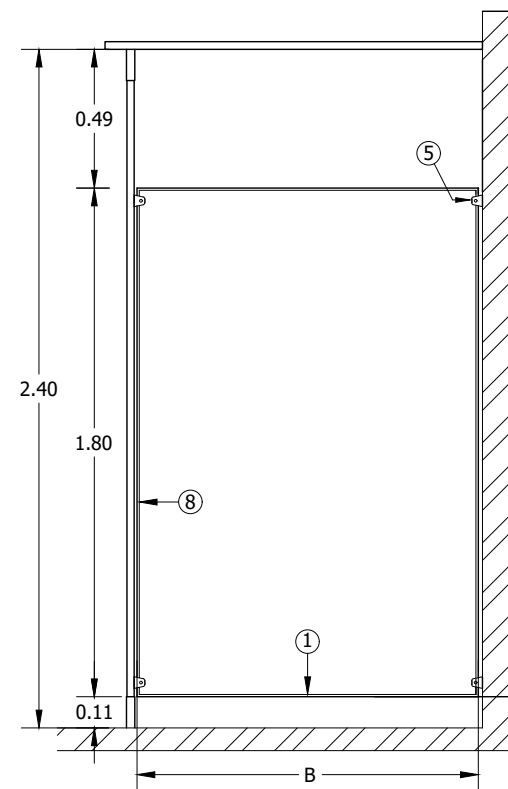
VISTA LATERAL
