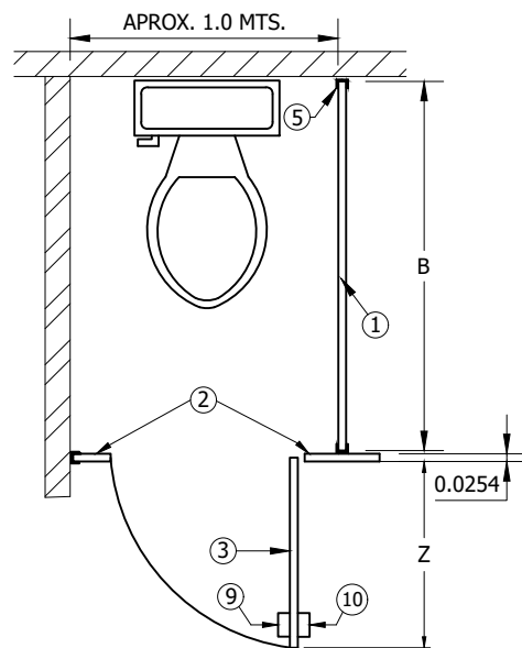
VISTA SUPERIOR
